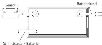
Abb. 8: Anschlusschema Schnittstelle RS485
