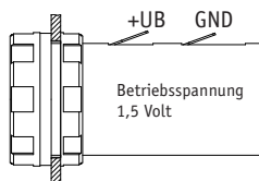
Abb. 9: Anschluss des Batteriefaches
